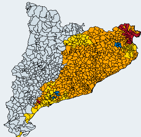
Estado sequía en septiembre de 2023
