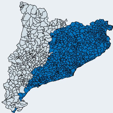
Estado sequía en enero de 2021
