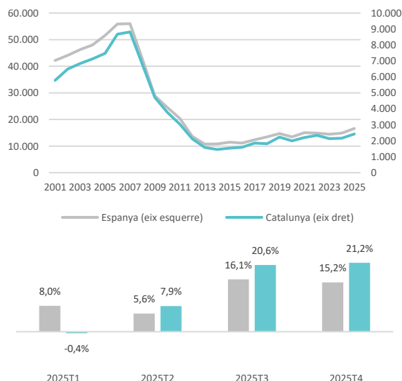
Figura 6. Evolució del consum de ciment en milers de tones a Espanya i Catalunya. Variacions interanuals del consum aparent de ciment durant el 2025 a Espanya i Catalunya
